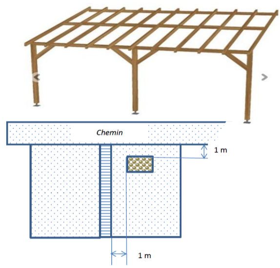
Plan N° 02 / Pavillon avec pergola sans annexe à outils / Franco Criscione, le 28.12.2020
